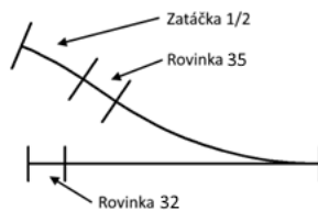
Výhybka pro klasické nádraží
